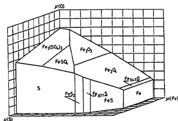
図1 Fe-O-S系高温化学ポテンシャル図 23)
