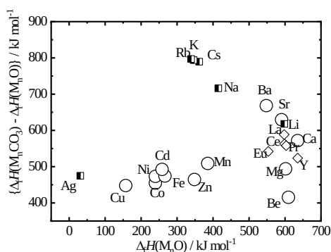
図 31 酸化物の生成エンタルピーに対してプロットした炭酸塩と酸化物のエンタルピー
